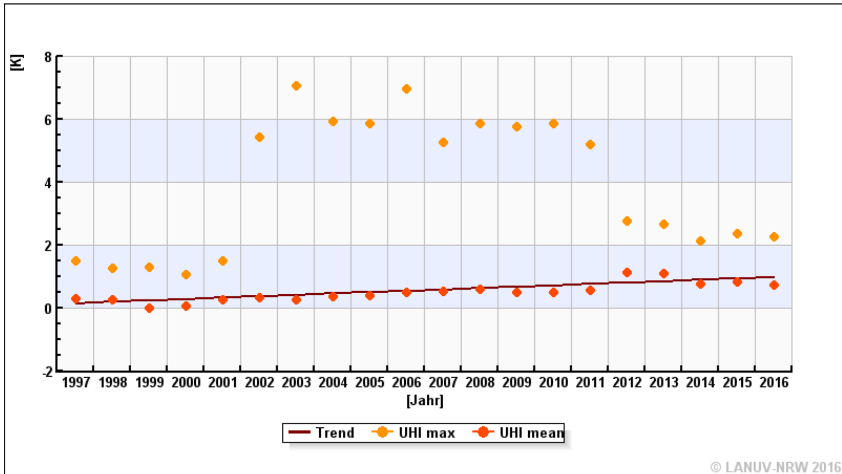
Abb.: Wärmeinselintensität Bochum (Klimafolgenmonitoring Landesamt für Natur, Umwelt und Verbraucherschutz Nordrhein-Westfalen) (Urban Heat Island = UHI)
